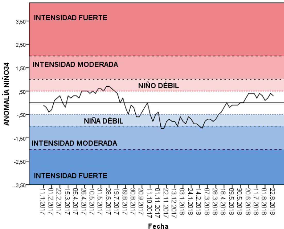
Gráfica N°2. Anomalías semanales de temperaturas de la superficie del mar (ATSM) Observadas en la región Niño34 hasta la semana centrada el 22 de agosto de 2018.
