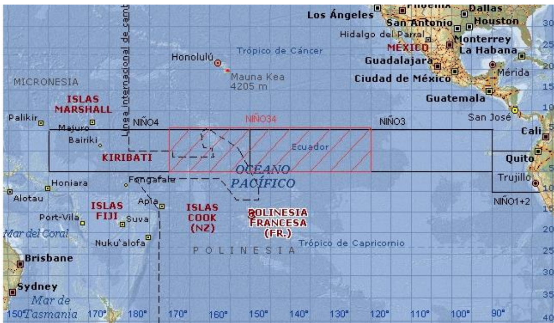
Gráfica N°1. Regiones de medición de la temperatura de la superficie del mar (TSM) en el pacífico ecuatorial. [Tomado y modificado de: http://www.cpc.ncep.noaa.gov/products/analysis_monitoring/lanina/enso_evolution-status-fcsts-web.pdf ].
