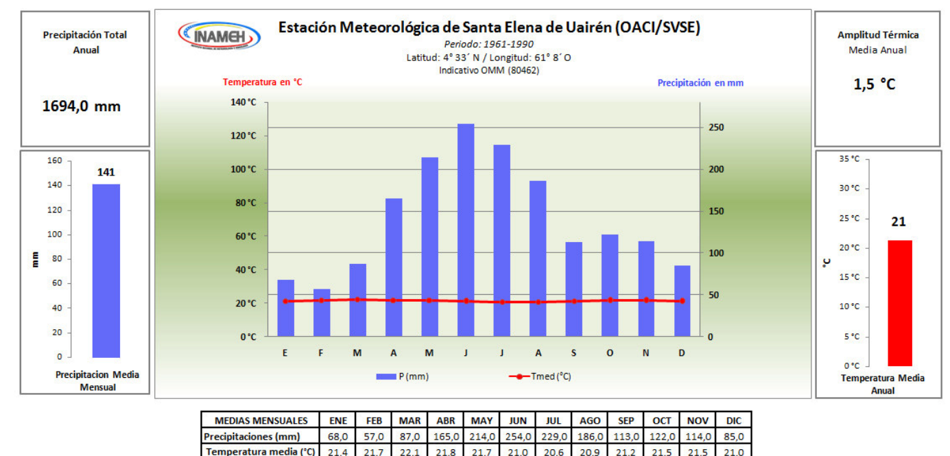
Climograma de la Estación Meteorológica de Sta. E. de Uairén, Estado Bolívar –Venezuela. Fuente: Servicio de Meteorología de la Aviación Militar Bolivariana
