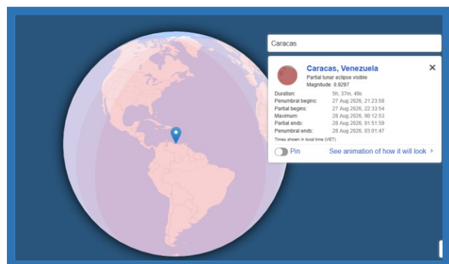
Figura 19. Eclipse Parcial de Luna.
