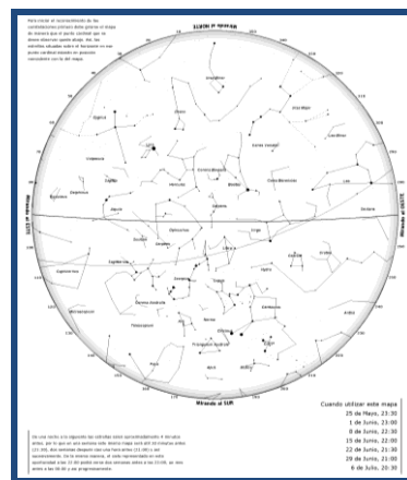
Figura 26. Cielo de Junio
