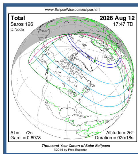
Figura 17. Eclipse Total de Sol.12 de Agosto 2026 Saros 126.
