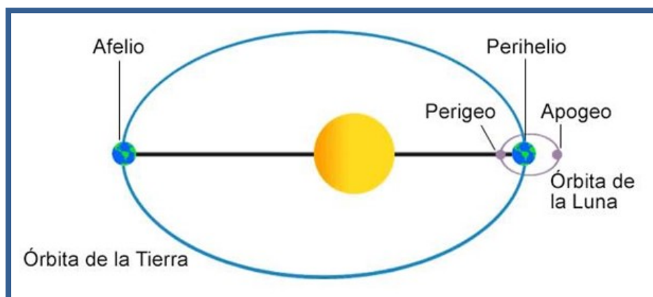
Figura 1. Fenómenos Geocéntricos
