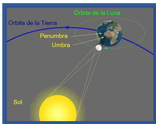
Figura 7. Eclipses Solares
