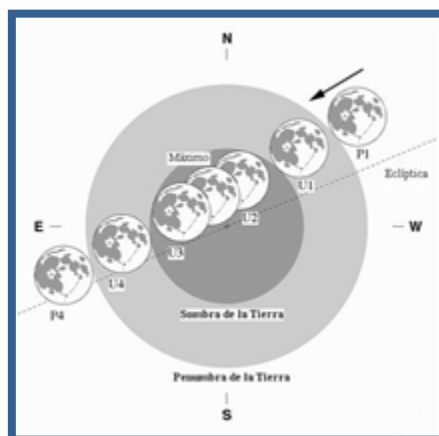
Figura 5. Eclipses Lunares
