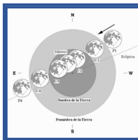
Figura 2. Eclipses Lunares
