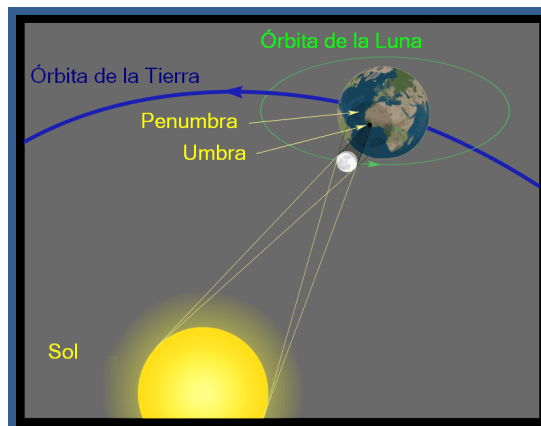
Figura 3. Eclipses Solares
