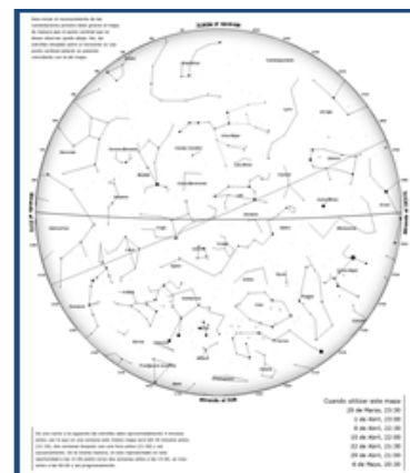
Figura 19. Cielo de Abril.
