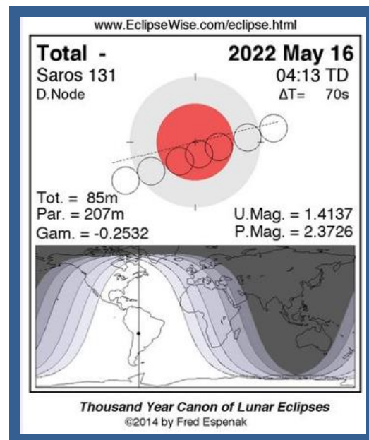
Figura 9. Eclipse Total de Luna. Saros 131.
