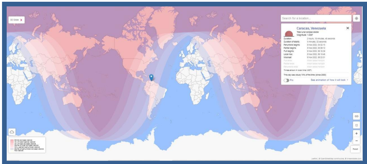
Figura 13. Eclipse Total de Luna 08 de Noviembre de 2022.
