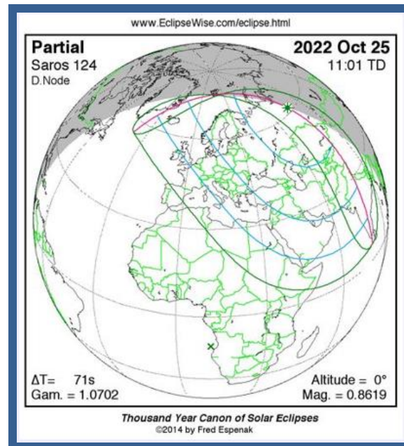
Figura 12. Eclipse Parcial de Sol 25 Octubre 2022. Saros 124.
