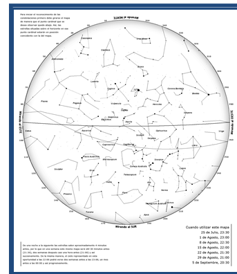
Figura 23. Cielo de Agosto
