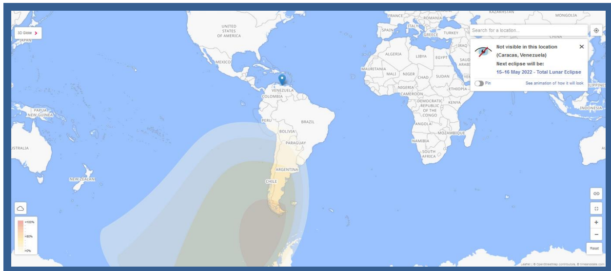
Figura 4. Eclipse Parcial de Sol.
