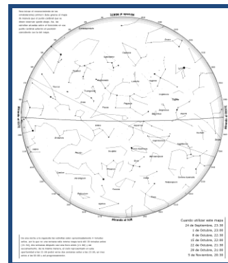
Figura 25. Cielo de Octubre
