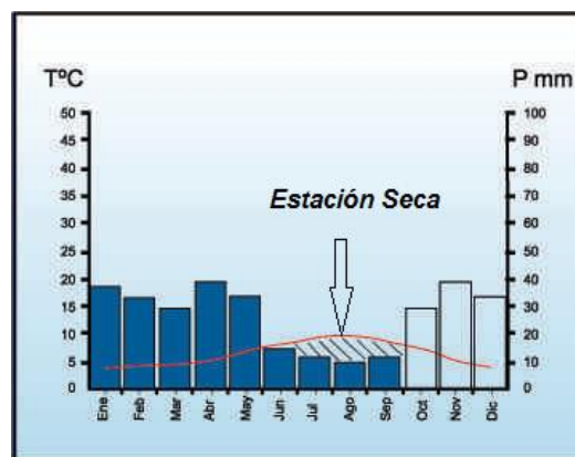
Figura 28. Ejemplo de un climograma donde se muestra la Estación Seca de un determinado lugar
