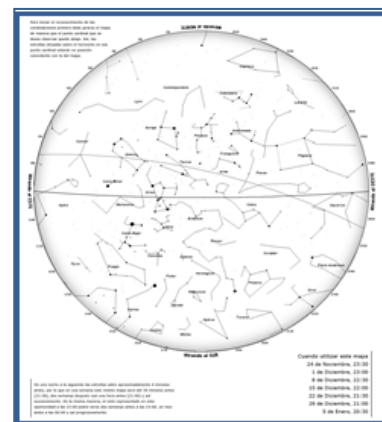
Figura 27. Cielo de Diciembre
