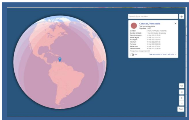
Figura 8. Mapa Eclipse Total de Luna 16 Mayo 2022.
