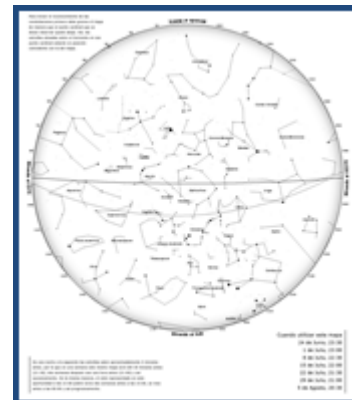
Figura 22. Cielo de Julio
