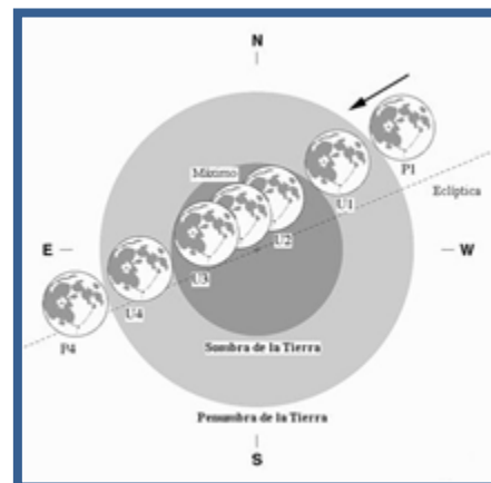
Figura 2. Eclipses Lunares
