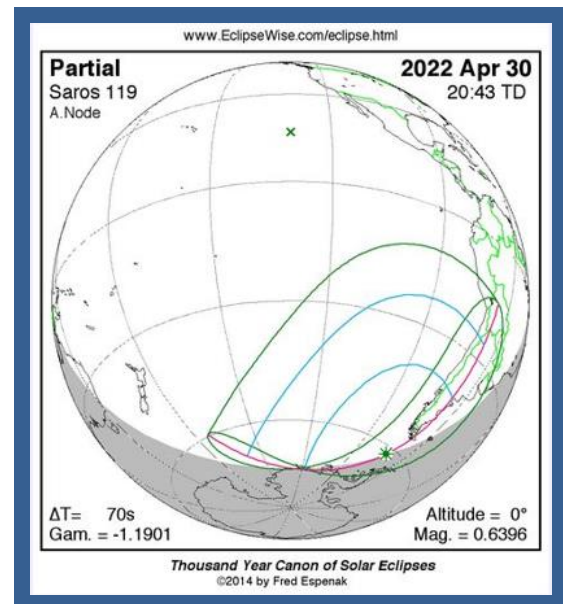
Figura 6. Eclipse Parcial de Sol. Saros 119.
