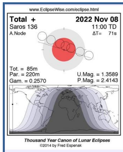
Figura 15. Mapa Eclipse Total de Luna. Saros 136.
