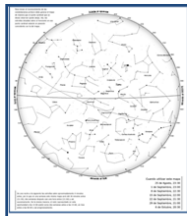
Figura 24. Cielo de Septiembre
