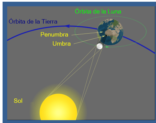
Figura 3. Eclipses Solares
