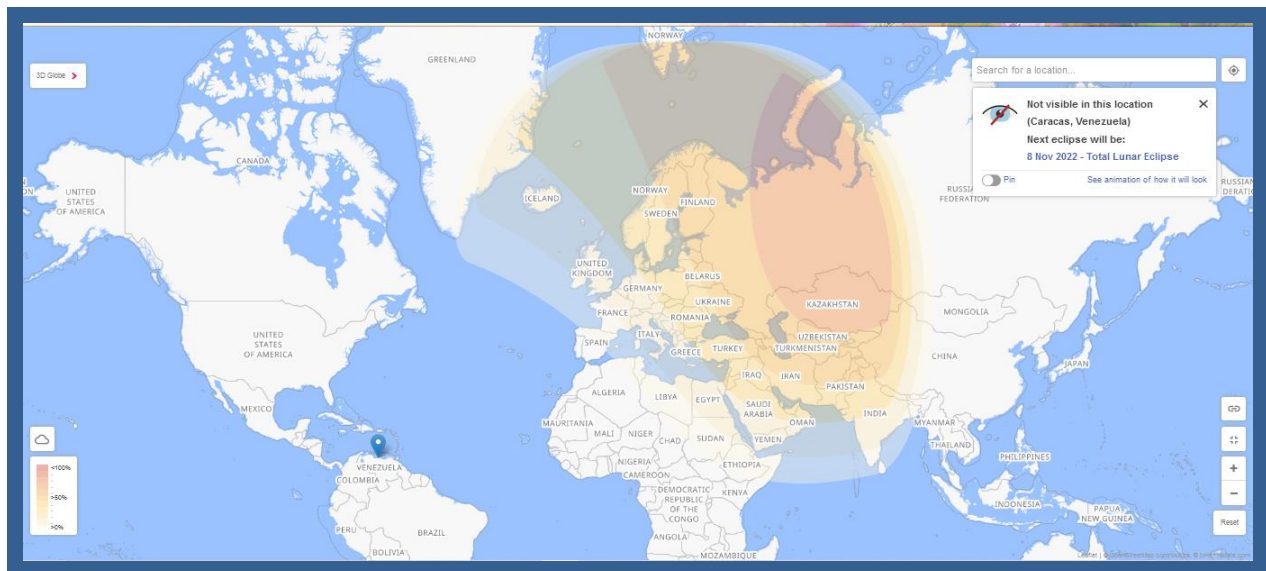
Figura 10. Eclipse Parcial de Sol 25 de Octubre 2022.
