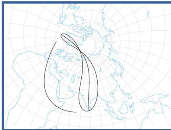
Figura 11. Mapa Eclipse Parcial de Sol.
