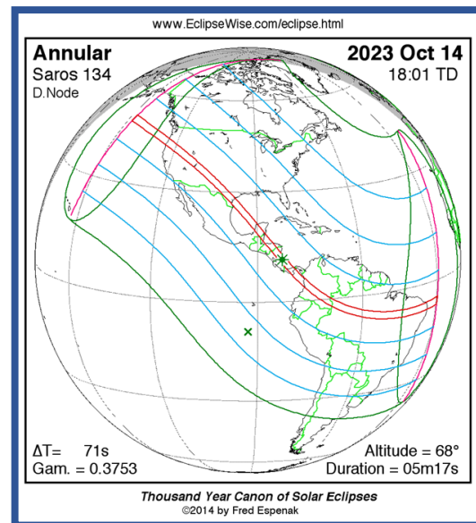
Figura 12. Eclipse Anular de Sol 14 Octubre 2023. Saros 134.
