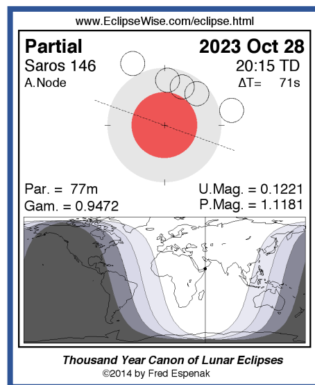
Figura 15. Mapa Eclipse Parcial de Luna. Saros 146.
