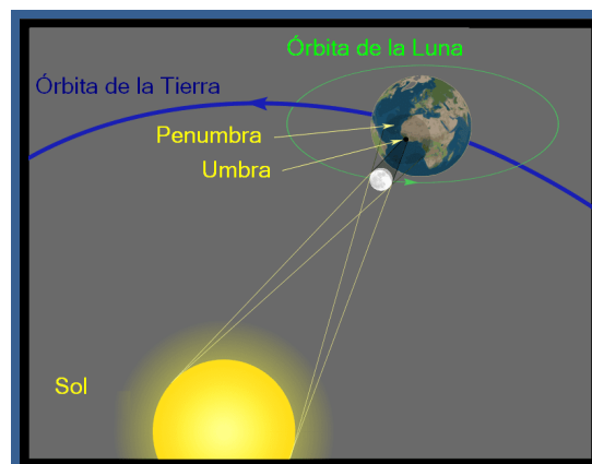
Figura 3. Eclipses Solares
