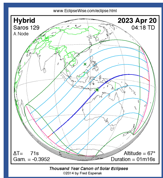
Figura 6. Eclipse Híbrido de Sol. Saros 129.
