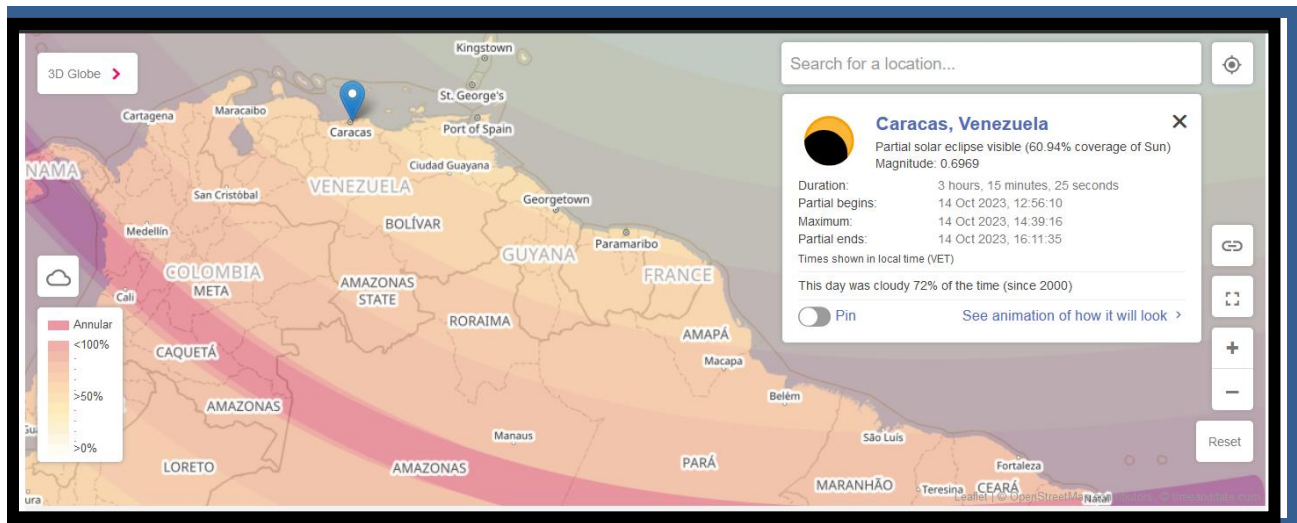
Figura 10. Eclipse Anular de Sol 14 de Octubre 2023.
