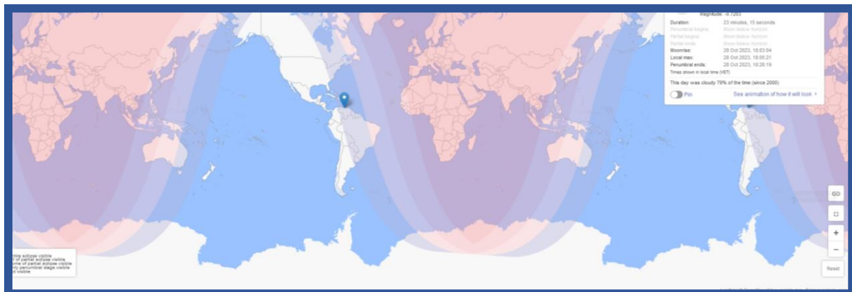
Figura 13. Eclipse Parcial de Luna 28 de Octubre de 2023.
