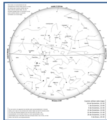
Figura 27. Cielo de Diciembre
