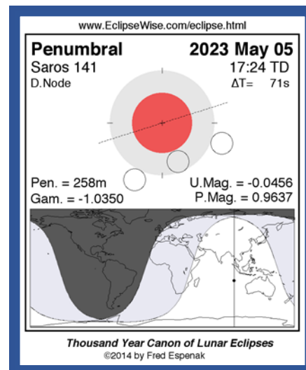
Figura 9. Eclipse Penumbral de Luna. Saros 141.
