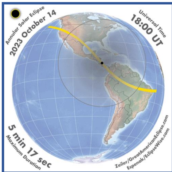
Figura 11. Mapa Eclipse Anular de Sol.
