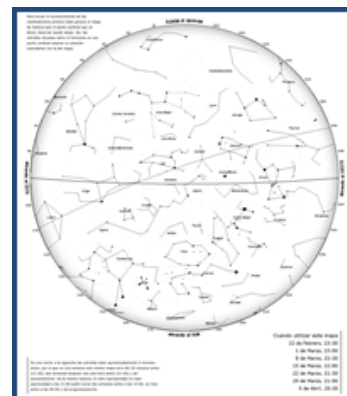
Figura 18. Cielo de Marzo
