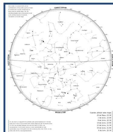
Figura 21. Cielo de Junio
