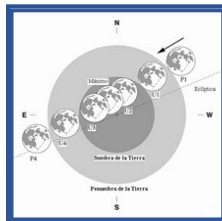
Figura 2. Eclipses Lunares
