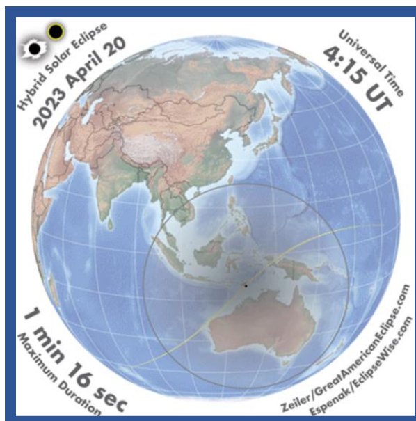
Figura 5. Mapa Eclipse Híbrido de Sol 20 Abril 2023.
