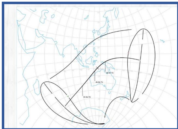
Figura 14. Eclipse Parcial de Luna.
